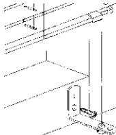
Wirebeslag ved veggfeste
