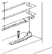
Wirebeslag ved takfeste
