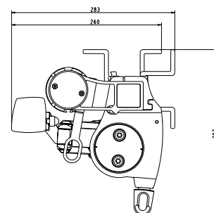
Norlux Flex med kombi vegg- og takfeste
