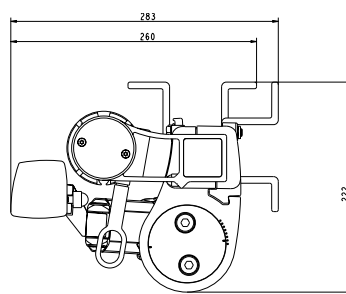
Norlux med kombi vegg- og takfeste
